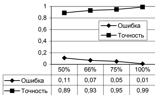
Рис. 5. Оценка точности обученного анализатора.
