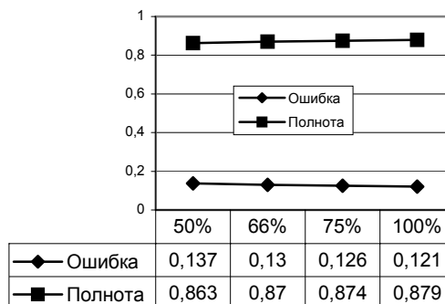
Рис. 6. Оценка полноты обученного анализатора.
