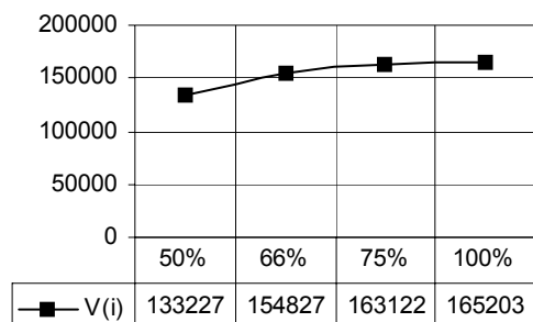
Рис. 2. Зависимость объема словаря обученного анализатора от объема обучающей выборки.
