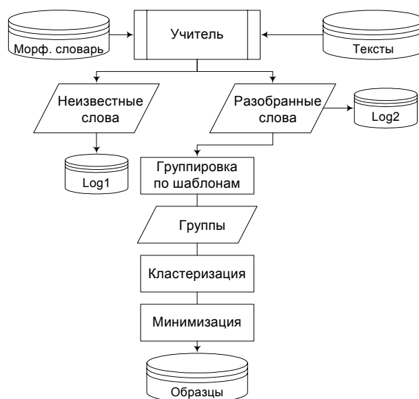
Рис. 1. Функциональная схема обучения.
