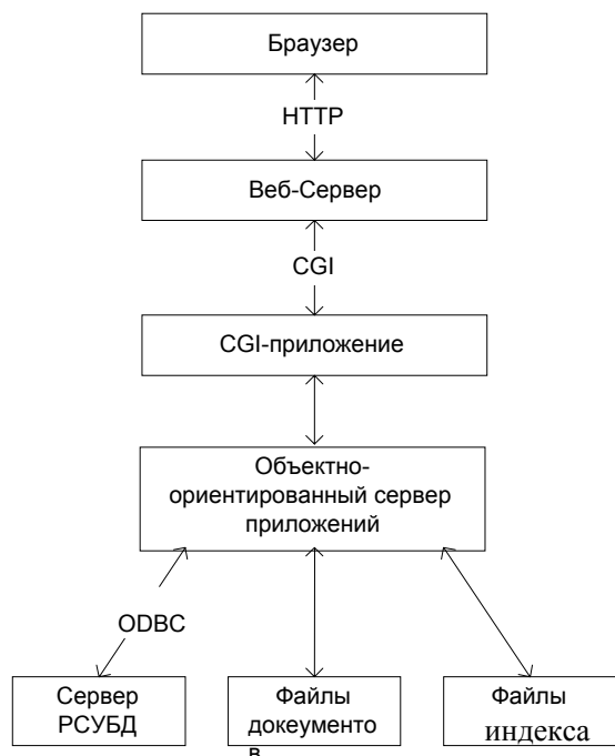
Рис. 2. Новая трехзвенная архитектура T-Libra
